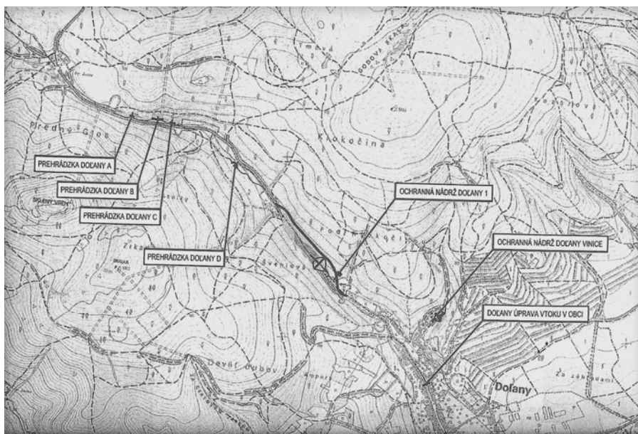
Projektované rozmiestnenie jednotlivých vodozádržných objektov.
