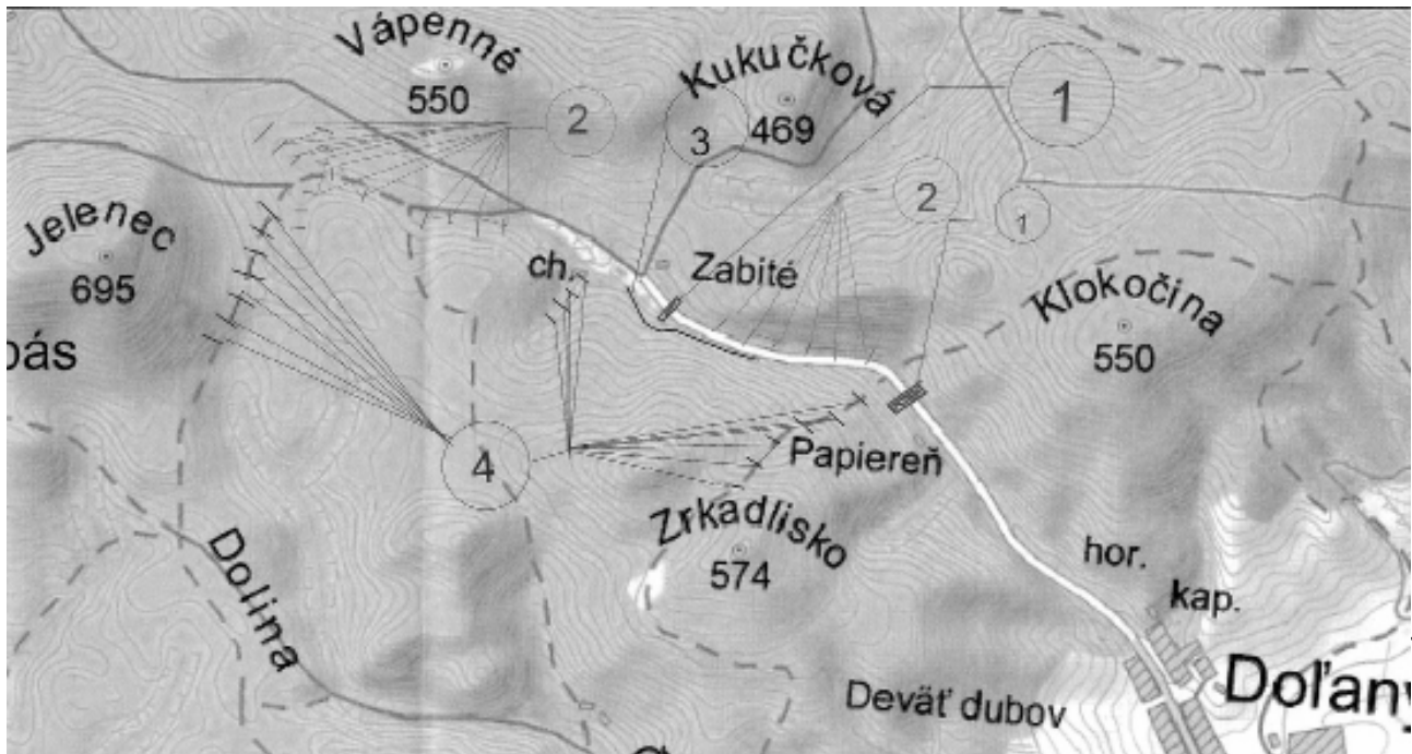
Legenda k obrázku: 1. Prehrádzky; 2. Garnisáže; 3. Zasakovací pás; 4. Odrážky
